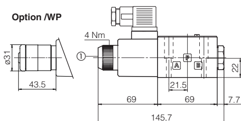
DHE-06(AC)
